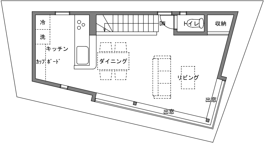
3階平面図 1/100
