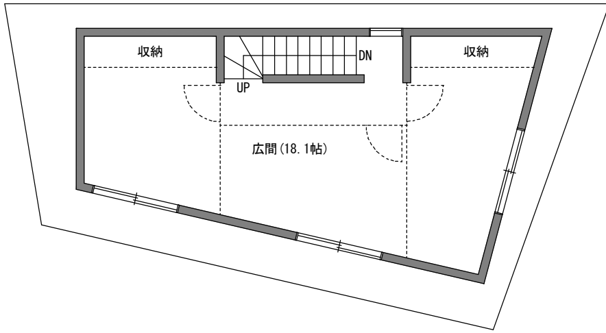
2階平面図 1/100
