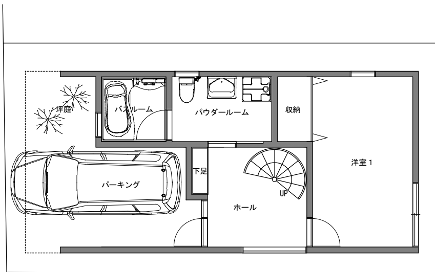
1階平面図 1/100
