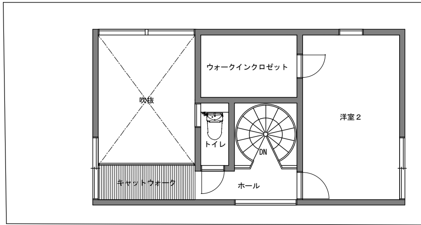
3階平面図 1/100
