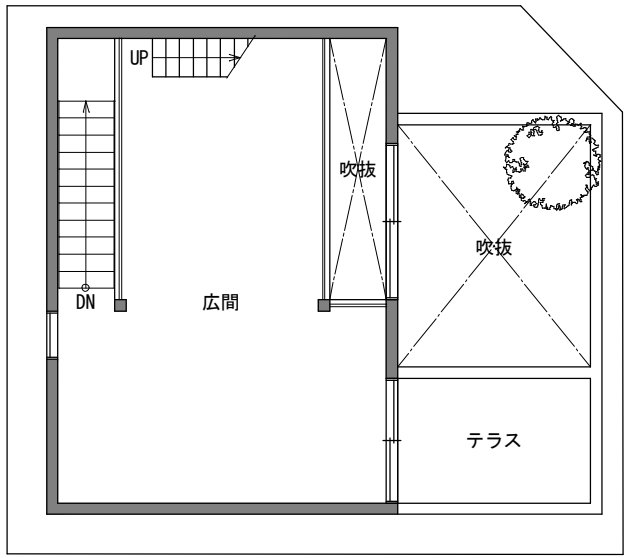
2階平面図 1/100
