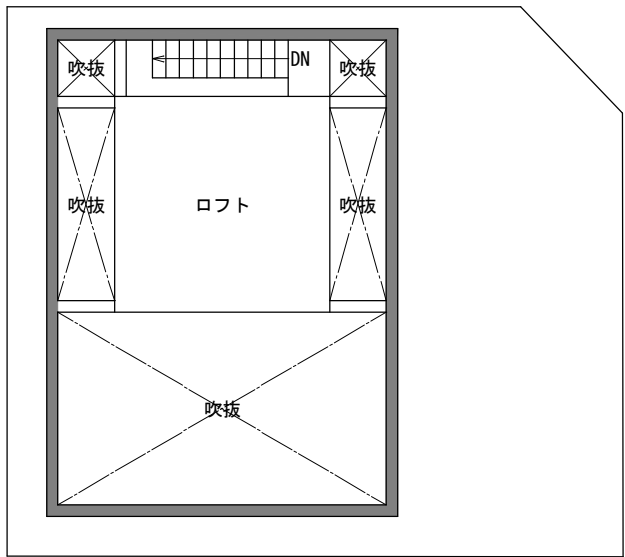
ロフト平面図 1/100
