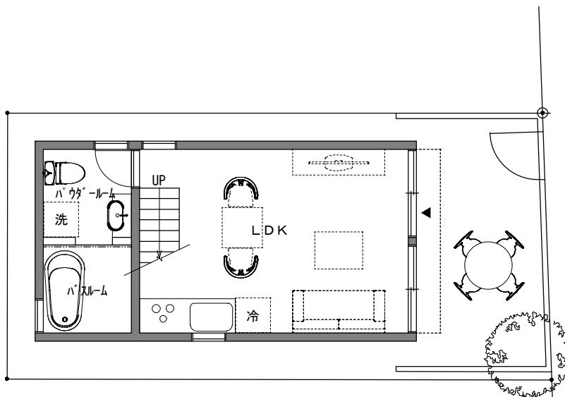
■ 1階平面図
