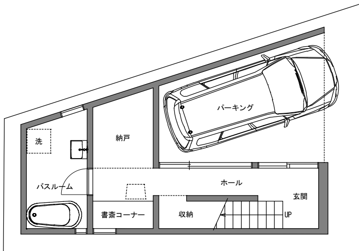
1階平面図 1/100
