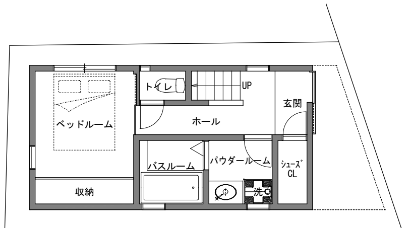
1階平面図 1/100
