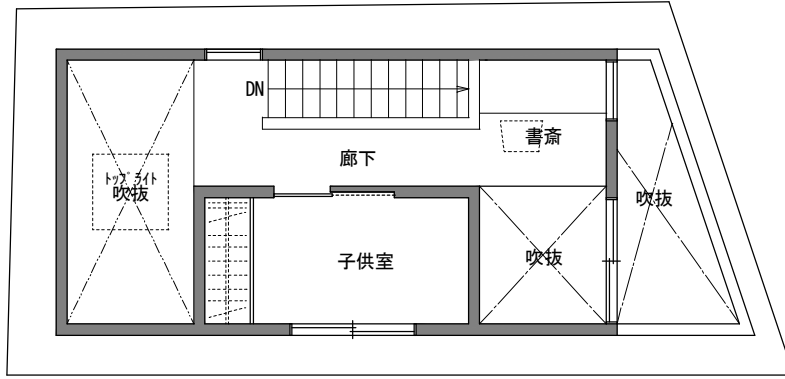
3階平面図 1/100
