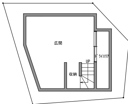
地下1階平面図 1/100
