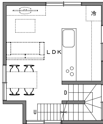
2階平面図 1/100
