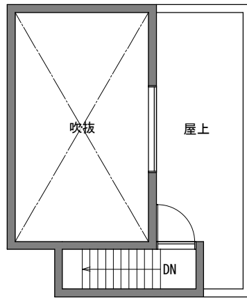
屋上平面図 1/100
