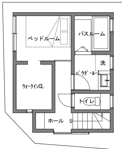
1階平面図 1/100
