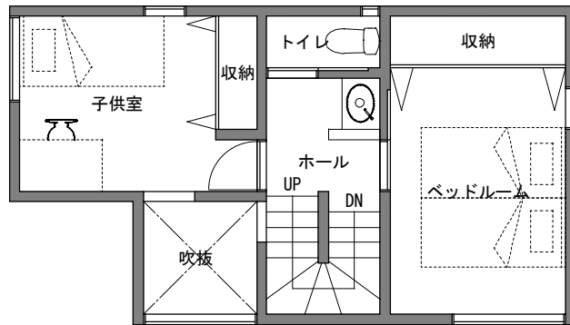
2階平面図 1/100
