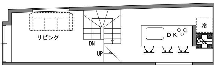
2階平面図 1/100
