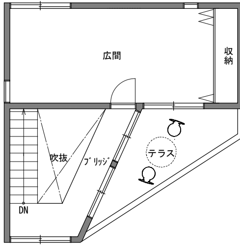
3階平面図 1/100
