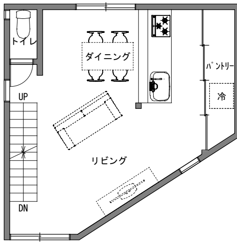
2階平面図 1/100
