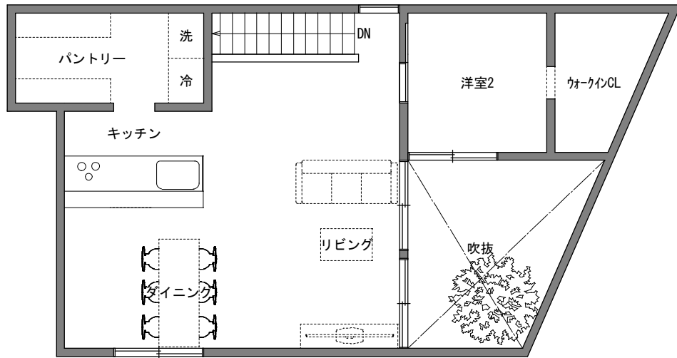
2階平面図 1/100
