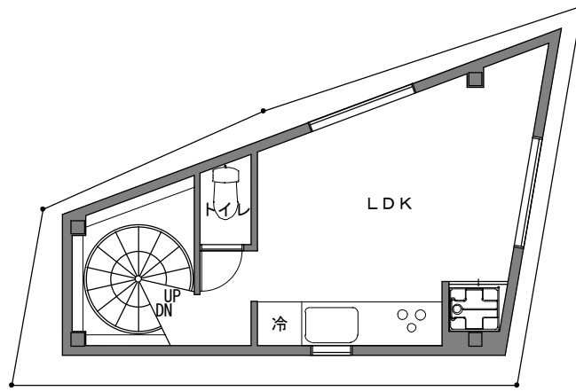
3階平面図 1/100
