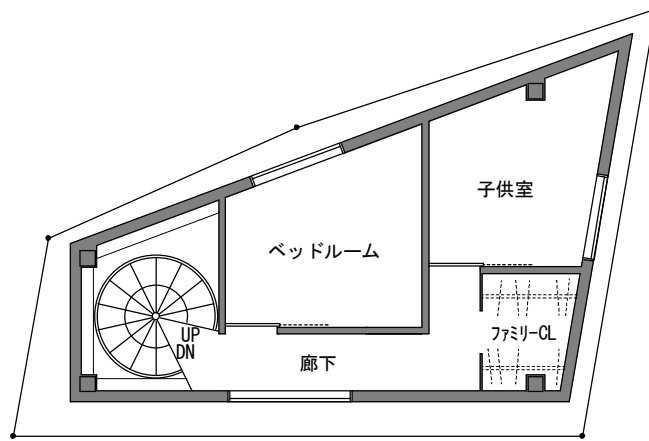
2階平面図 1/100
