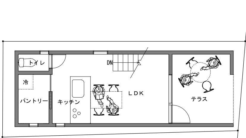
■ 1階平面図
