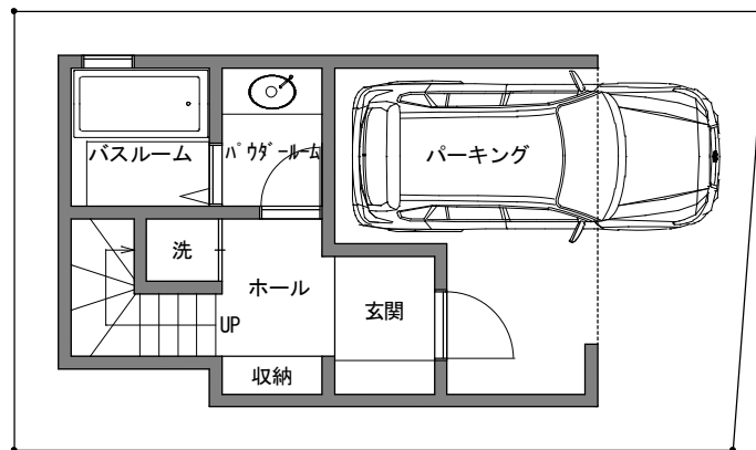
1 階平面図 1/100
