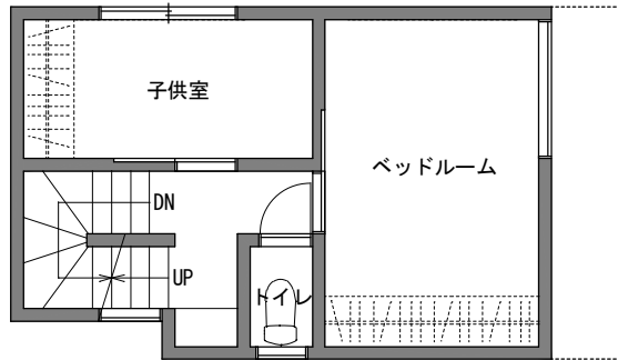
2 階平面図 1/100
