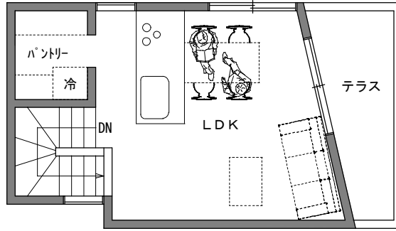
3 階平面図 1/100
