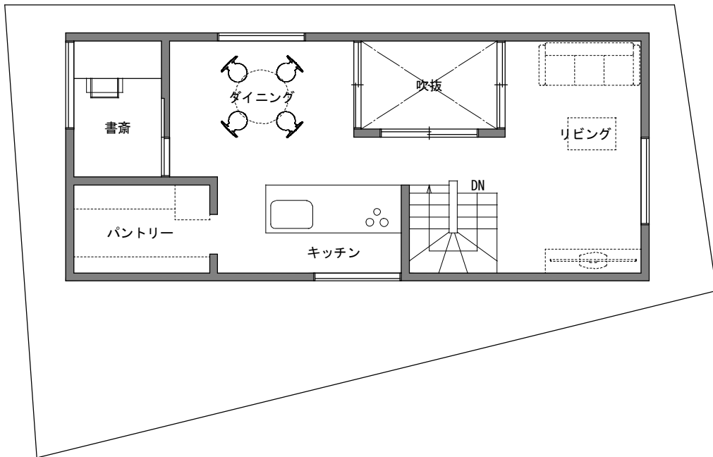
2階平面図 1/100
