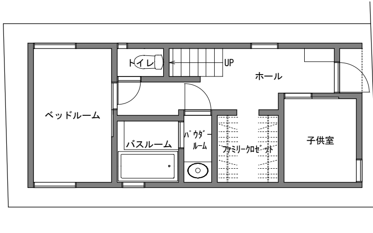
1階平面図 1/100
