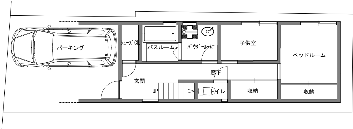
1階平面図 1/100
