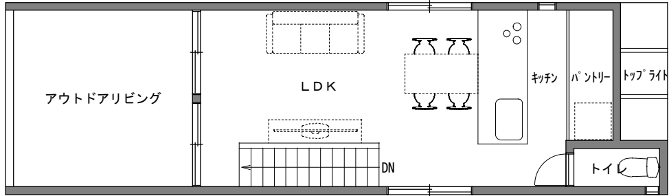
2階平面図 1/100
