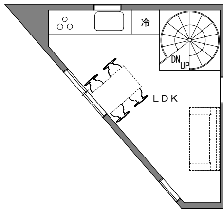
2階平面図 1/100
