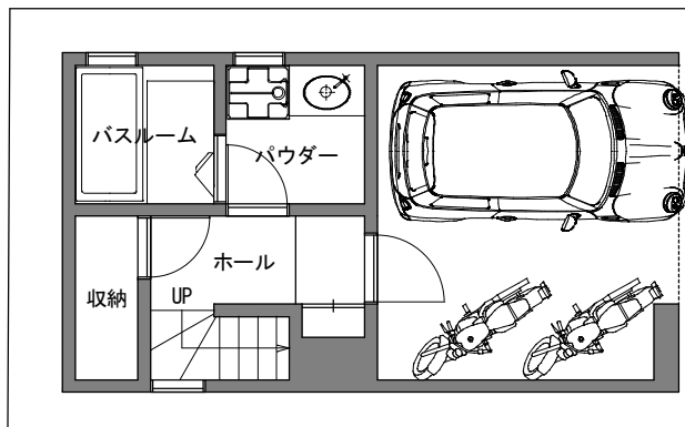
1階平面図 1/100
