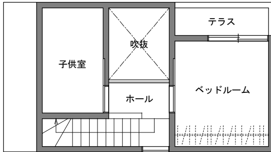
3階平面図 1/100
