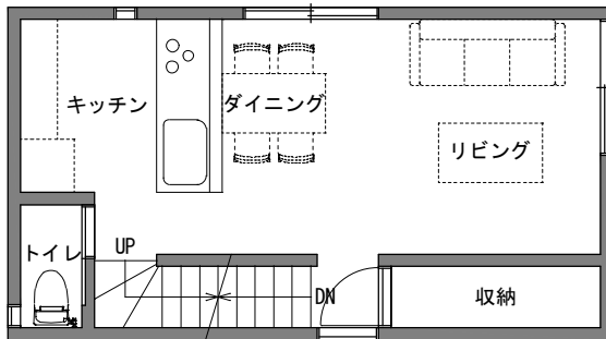
2階平面図 1/100
